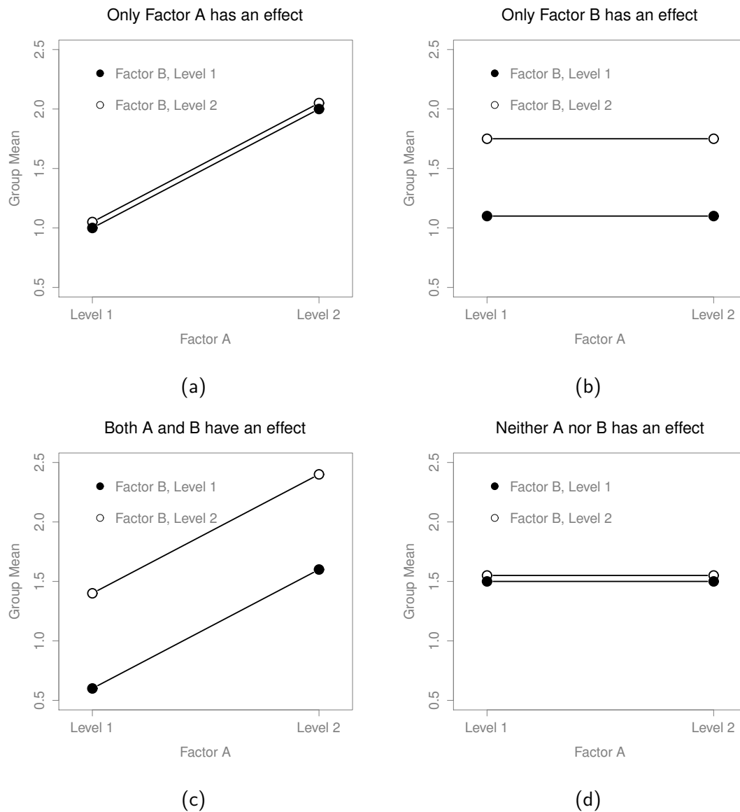
Figure1.5 交互作用のない2×2要因の分散分析における4つの出力。パネル(a)は要因Aの主効果があり、要因Bの主効果がない場合。パネル(b)は要因Aの主効果がなく、要因Bの主効果がある場合。パネル(c)は要因A、要因Bのどちらの主効果もある場合。パネル(d)はどちらの要因の主効果もない場合。
